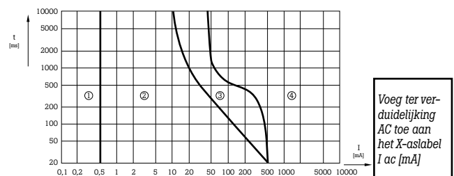
Afb. 1: effecten van AC-stroom (voor RMS-waarden van 50 Hz tot 60 Hz)
