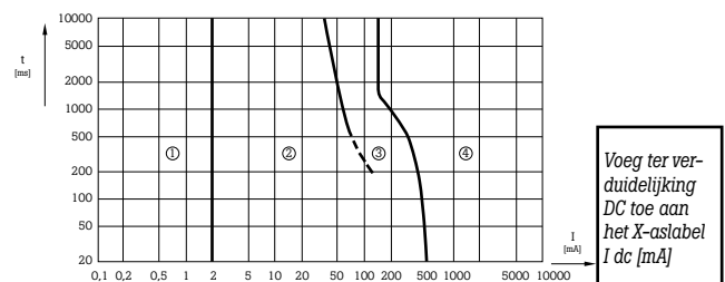
Afb. 2: effecten van DC-stroom
