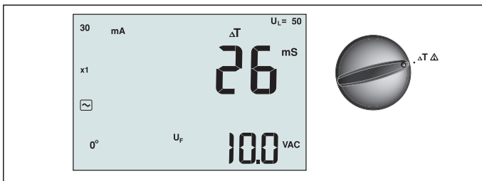
Abbildung 16. Anzeige der FI/RCD-Auslösezeit / Schalterstellung / Anschlussbelegung
